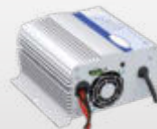
Chargeur de batterie 12 V / 25 A / 300 W
